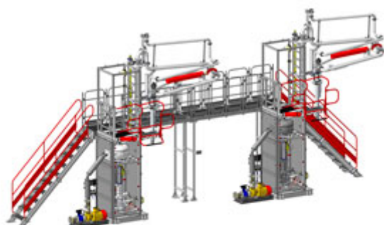
АСН-8ВГ НОРД Ду100 2/2 (КМ-СМФ-300) ХЛ2
