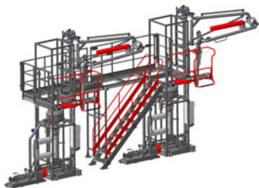
АСН-8ВГ Модуль Ду100 2/2 (КМ-СМФ-300) У2
