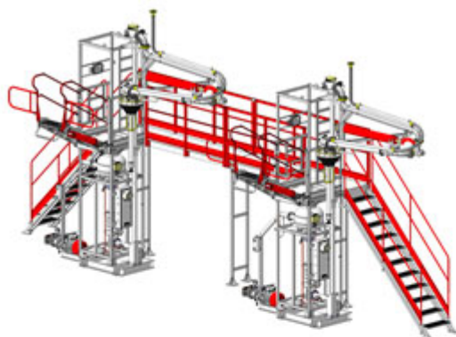
АСН-8ВГ Модуль Ду100 2/2 (КМ-ППВ) У2
