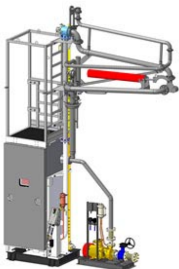
АСН-5ВГ Модуль Ду100 (КМ-ППВ) Х12
