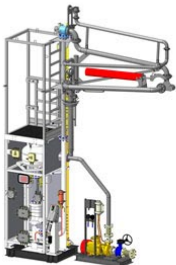
АСН-5ВГ Модуль Ду100 (КМ-ППВ) У2
