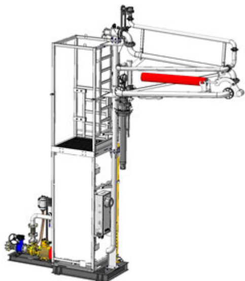
АСН-5ВГ НОРД Ду100 с насосным блоком
