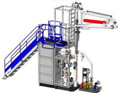
АСН-12ВГ модуль Ду100 (КМ – ППВ) У2 в комплекте с дозатором ввода присадок
