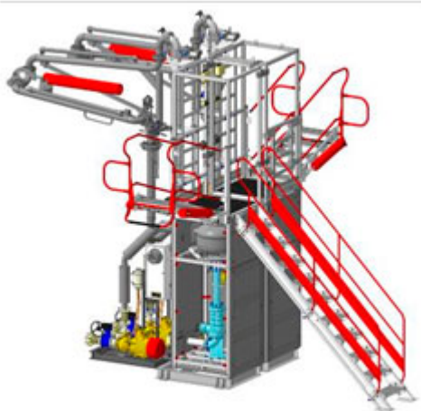
АСН-10ВГ НОРД Ду100 2/2 (КМ-ППВ)
