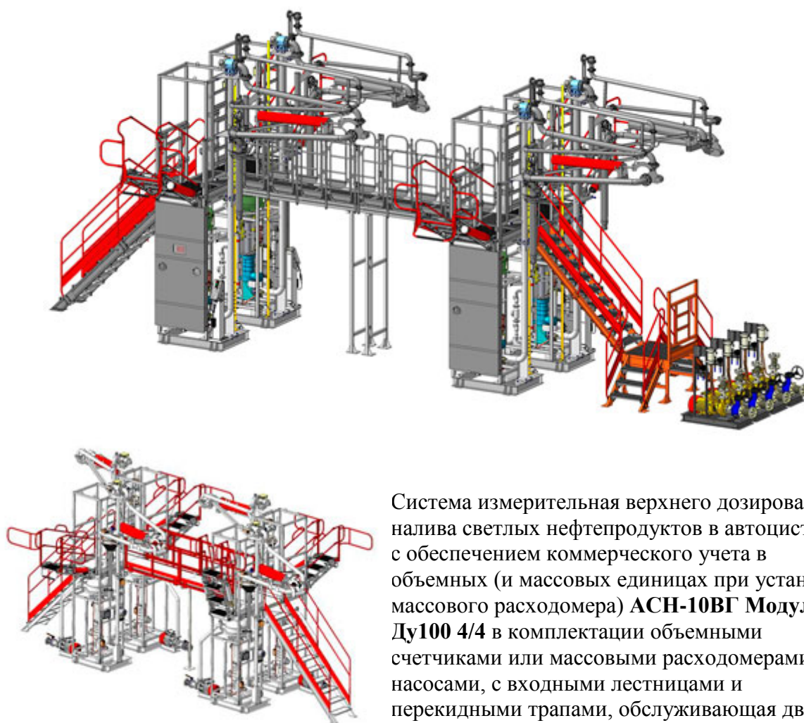
АСН-10ВГ Модуль Ду100 4/4
